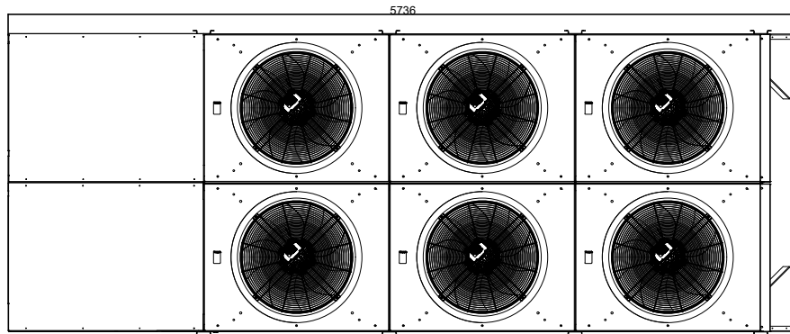
VISTA PLANTA
