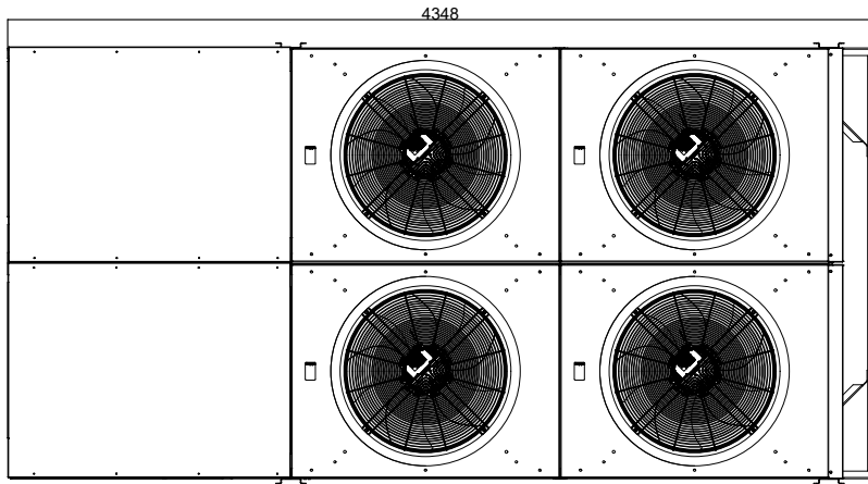
VISTA PLANTA
